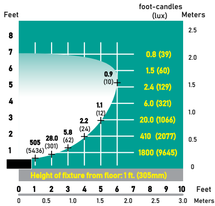
CS-LFL-01HE-LEDP8 Half Spread Photometrics
