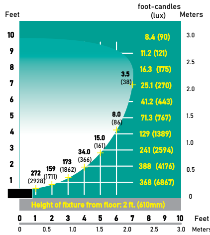
CS-LFL-01-LEDP8 Half Spread Photometrics
