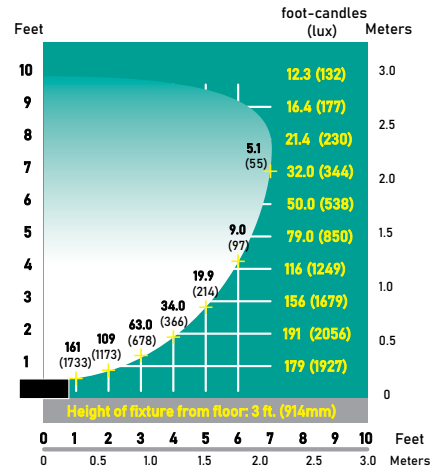
CS-LFL-01-LEDP8 Half Spread Photometrics
